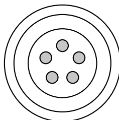
PRISE EURO CEE 32 400 V / 32 A Ø 65 mm
